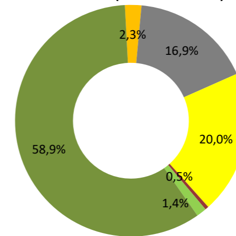
verbleibender Energieträgermix alle Produkte (außer Ökostrom)
