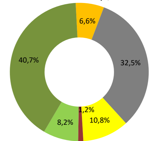
Zum Vergleich: Energieträgermix in Deutschland im Jahr 2022 (Quelle: BDEW)
